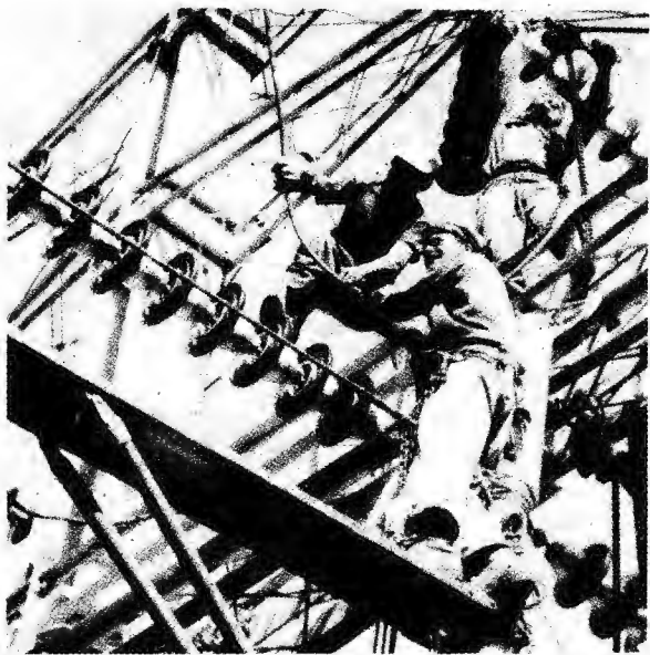
TECNICOS Y OBREROS ESTIRAN Y REVISAN UNO DE LOS CABLES: 35 KILOMETROS DE LARGO
