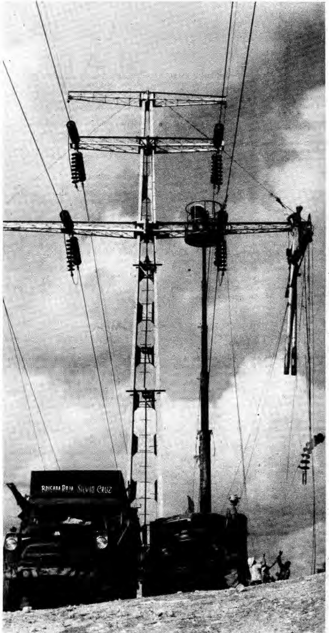
LOS TRABAJADORES ALZAN LOS AISLADORES DE PORCELANA, PARA SU INSTALACION EN LAS CRUCETAS
